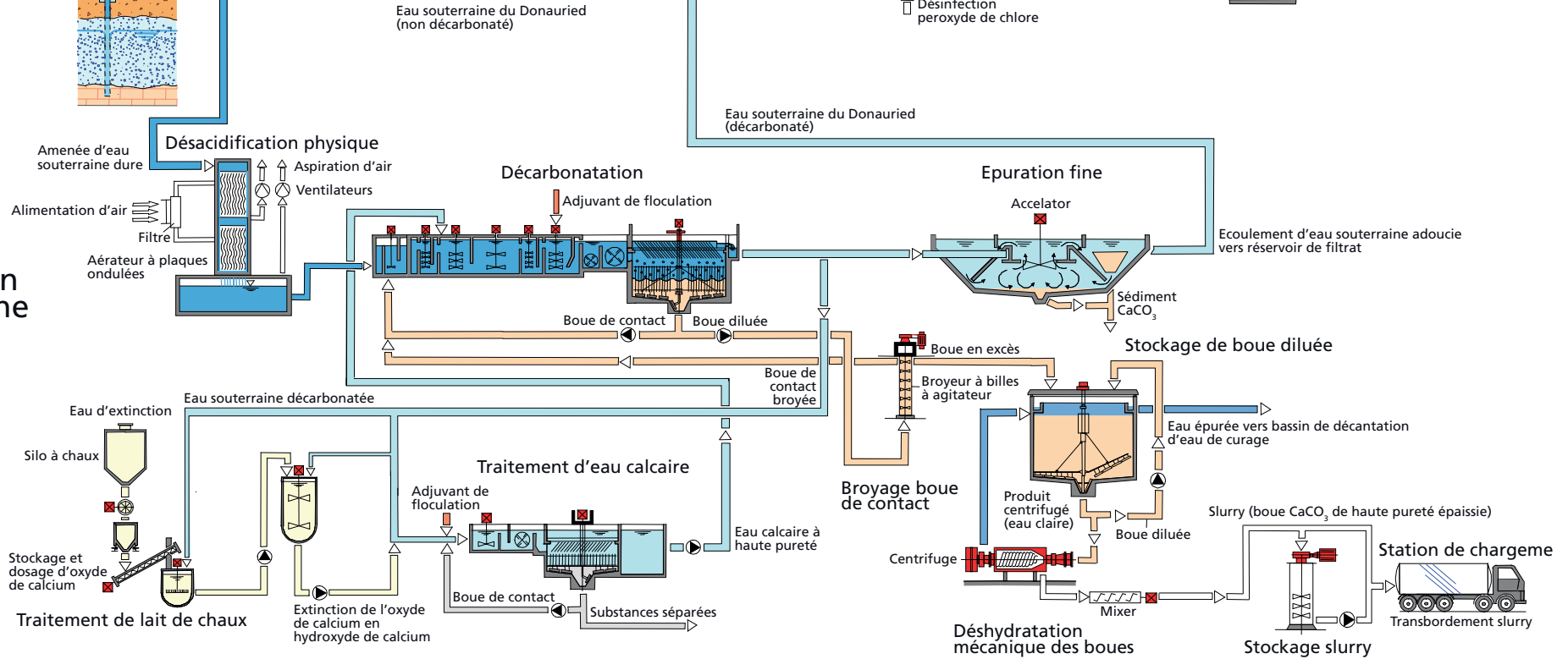
Schéma du procédé de traitement d'eau potable à la station hydraulique Langenau
